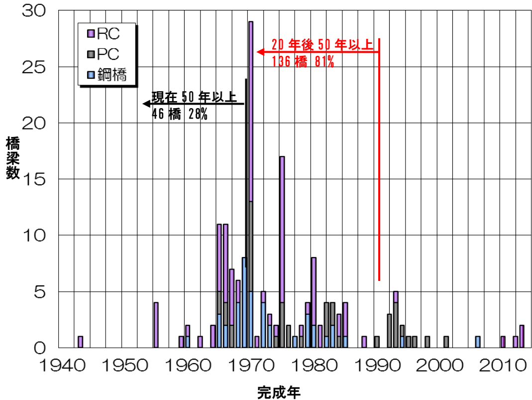
▲架設年・橋種別の橋梁数分布
