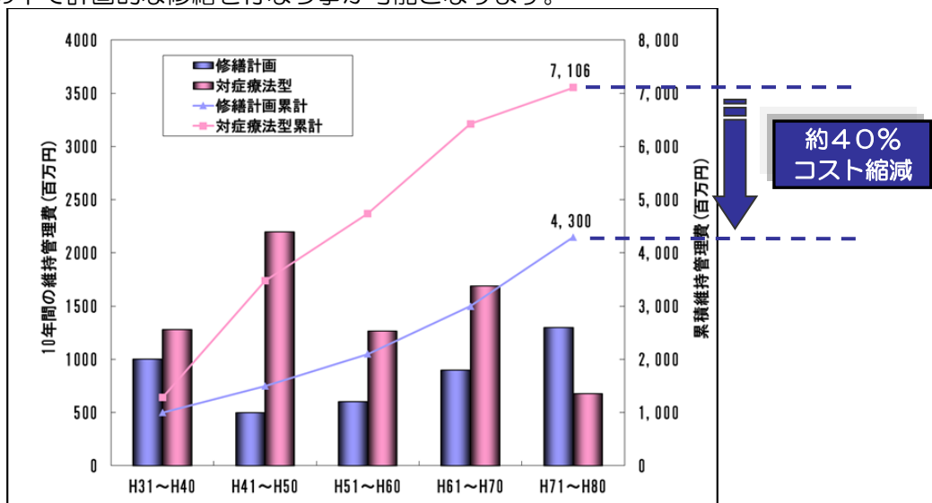
▲今後50年間の維持管理費の比較
