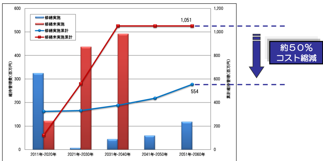
▲修繕実施による維持管理費縮減効果
