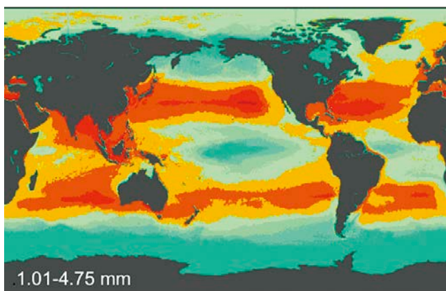
マイクロプラスチックの密度分布（モデル予測）
